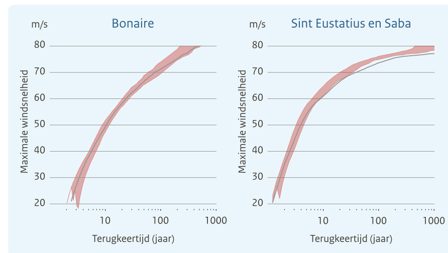
Figuur 30. Herhalingsperiodes van windsnelheden binnen 250 km van de BES-eilanden, nu (1980-2017, grijs) en in de toekomst (2015-2050, rood) bij het hoge uitstootscenario.
