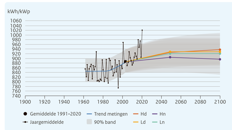
Figuur 37. Jaarlijkse energieopbrengst in Nederland van een standaard eenheid van zonnepanelen sinds 1965 tot 2022 en voor het toekomstige klimaat volgens de vier KNMI'23-klimaatsscenario's.
