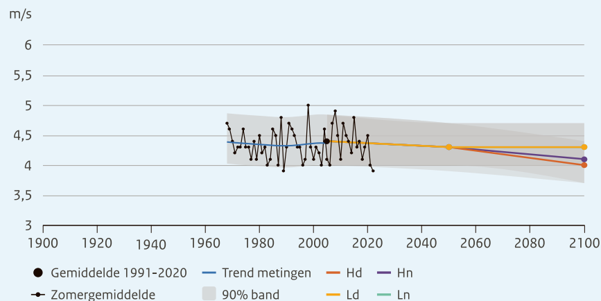
Figuur 21. Gemiddelde windsnelheid in de winter (links) en de zomer (rechts) op station Schiphol: waarnemingen (zwart) en de vier KNMI'23-klimaatscenario's (2050 en 2100).
