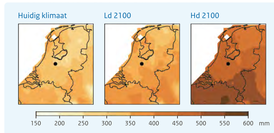
Figuur 18. Het maximale neerslagtekort in de 5% droogste jaren in het huidige klimaat en in de twee droge KNMI'23-klimaatsscenario's rond 2100. Zwarte stip: De Bilt (figuur 17).
