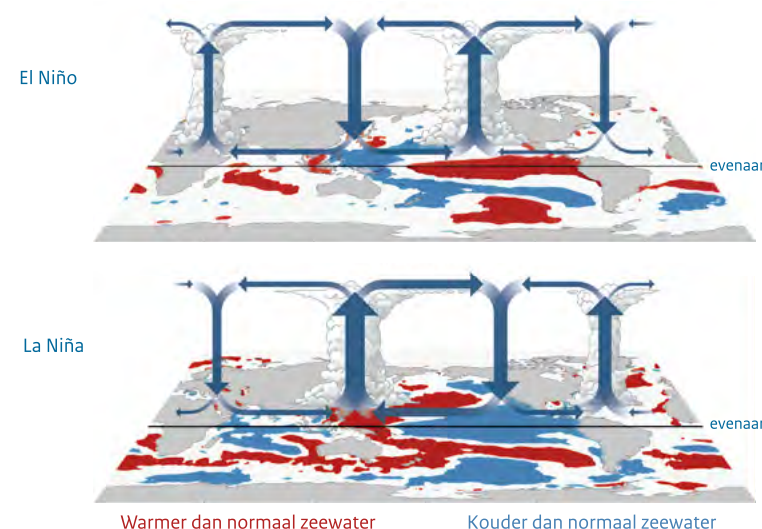
Figuur 46. Veranderingen van de wind rond de evenaar (Walker-circulatie) en zeevatertemperatuur tijdens El Niño (boven) en La Niña (onder). Bron: KNMI/NOAA.
