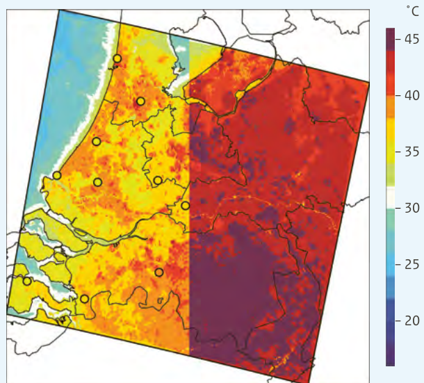
Figuur 11. Gemiddelde maximumtemperatuur op 24-26 juli 2019, uit waarnemingen (stippen) en regionale klimaatsimulaties voor het huidige klimaat (linkerhelft) en voor een 2°C warmer klimaat (rechterhelft).
