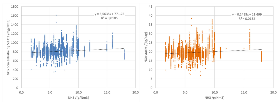
Figuur 23 : \text{NO}_x concentratie en vracht vs \text{NH}_3 concentratie in KO-gas bij schoorsteen 11
