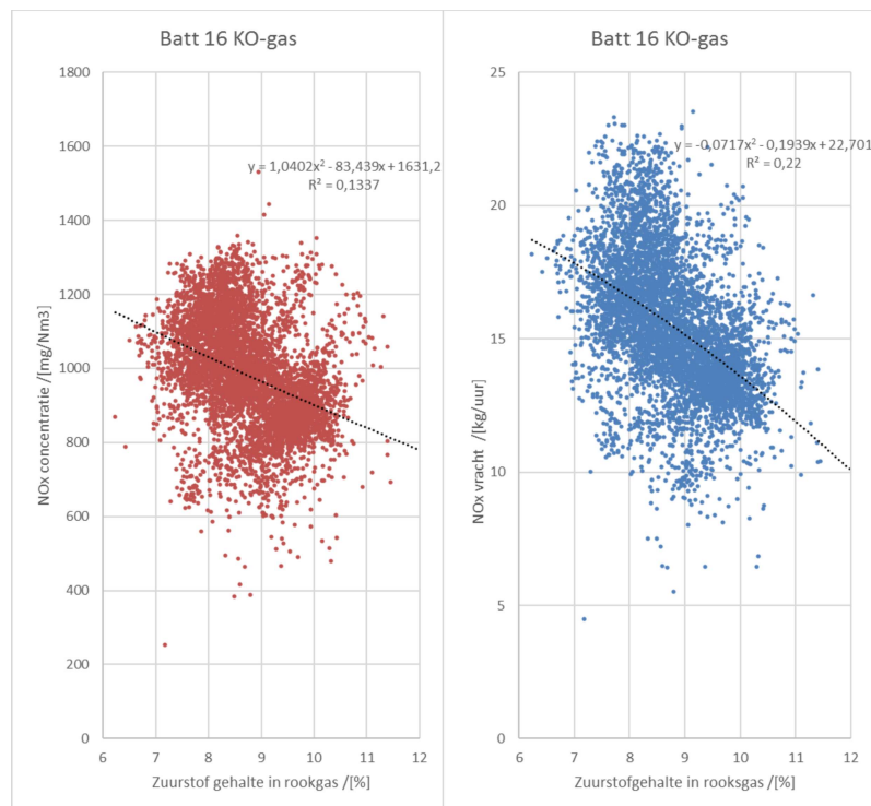
Figuur 29 : NO x concentratie en vracht vs het zuurstofgehalte in het rookgas van schoorsteen 13 bij KO-gas stoken.
