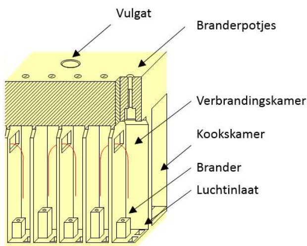
Figuur 8 : Doorsnede van een verbrandingswand
