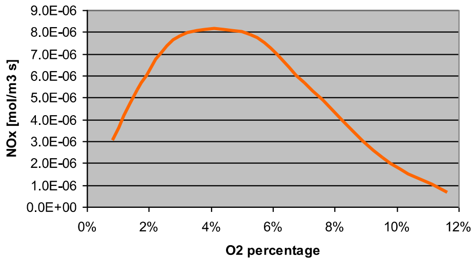
Figuur 3 : \text{NO}_x vormingssnelheid als functie van het zuurstofpercentage in de rookgassen
