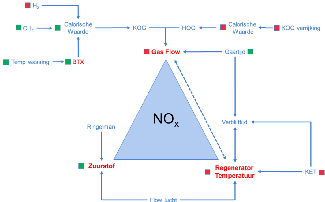
Figuur 5 : diagram met onderlinge verbondenheid van de procesparameters die NO x beïnvloeden.
