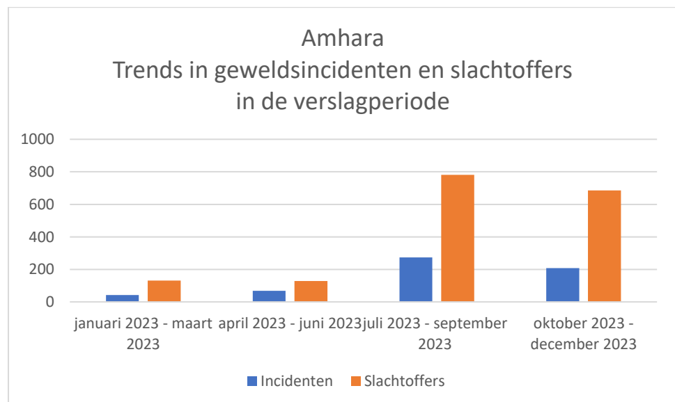
Afbeelding 11: Amhara – Trends in geweldsincidenten en dodelijke slachtoffers gedurende de verslagperiode december 2022-december 2023. Bron: ACLED.
